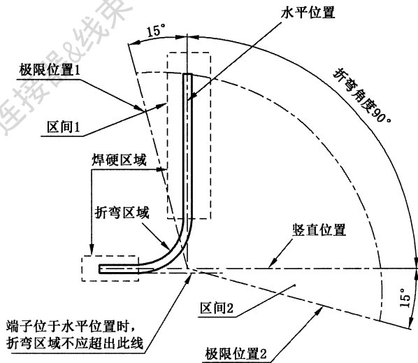
图 C.1 折弯测试示意图
