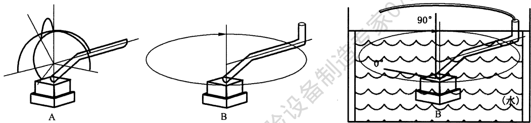
图 A.1 动态密封测试示意图
