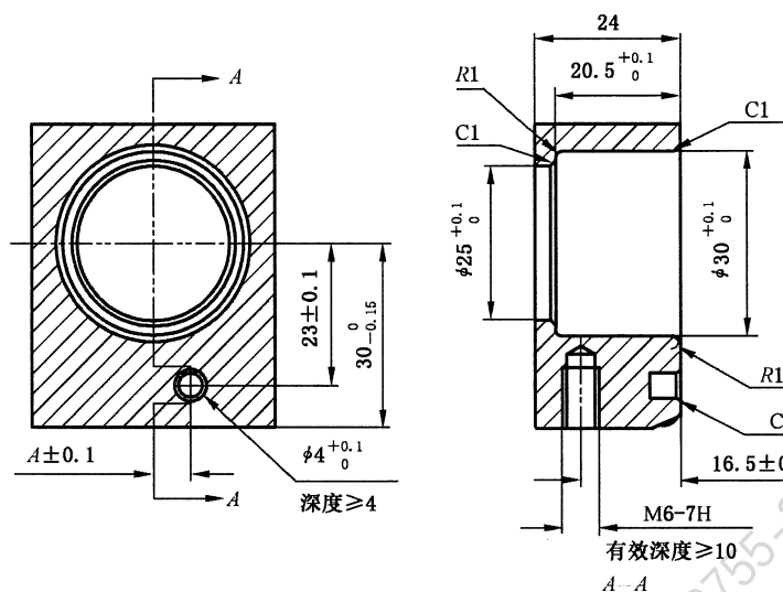
图 D.6 单芯集成式贯通连接器固定端安装尺寸
