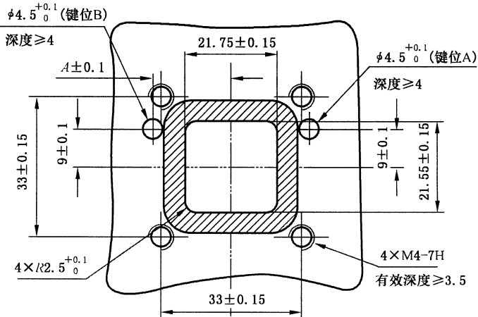
图 D.3 3 芯对插式小电流连接器固定端安装尺寸
